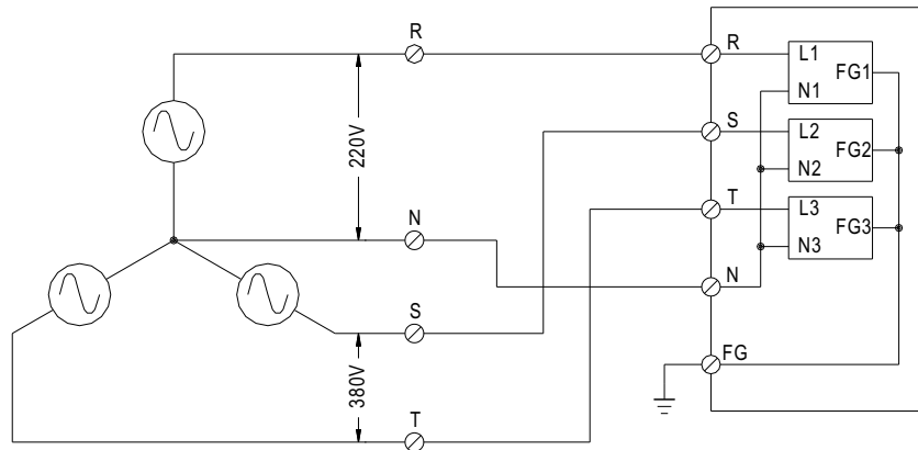
■ FIG. B: 3 φ 4W 220/380VAC SYSTEM
