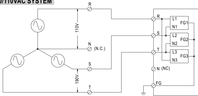
■ FIG. C: 3 φ 4W 190/110VAC SYSTEM
